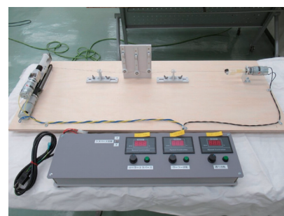
カーボンナノチューブ紡績装置<実験>
