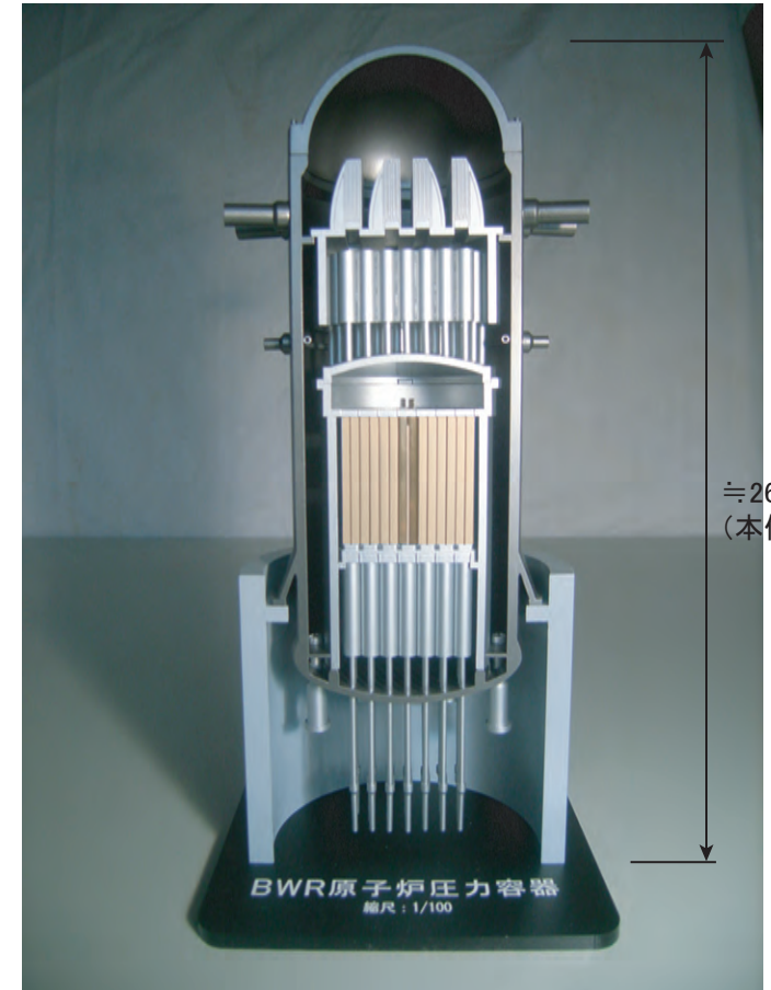
原子炉圧力容器蓋を載せて完成
